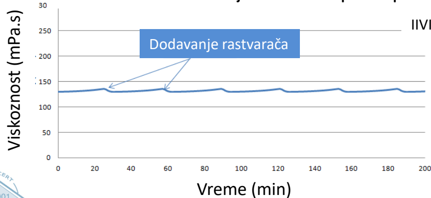
Kontrola viskoznosti dodavanjem rastvarača u procesu premazivanja
